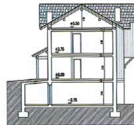
SEZIONE AA
