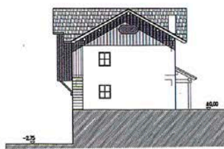
PROSPETTO EST
